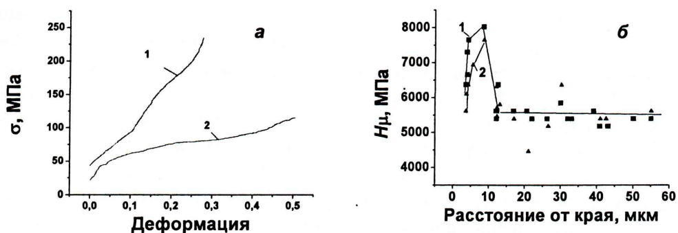
Рис. 3. Механические свойства стали AISI 304 (1) и Ст. 3 (2): а — кривые пластической деформации при сжатии; б — микротвердость в зависимости от расстояния от поверхности трения.
