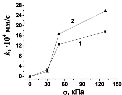
Рис. 4. Зависимость скорости линейного износа сталей AISI 304 (1) и Ст. 3 (2) по коксу в зависимости от приложенной нагрузки.
