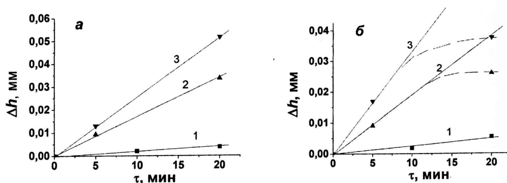
Рис. 2. Зависимости линейного износа Ст. 3 (а) и AISI 304 (б) от времени трения и нагрузки (кПа): 1 — 30; 2 — 50; 3 — 130.
